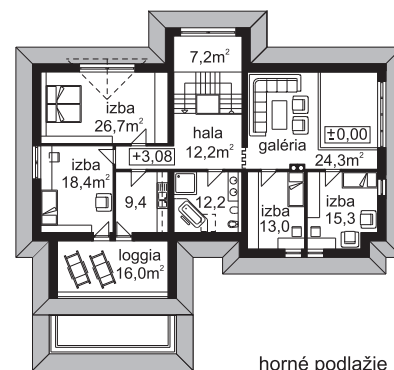
horné podlažie
