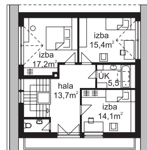
podkrovie
