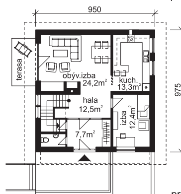
prízemie
