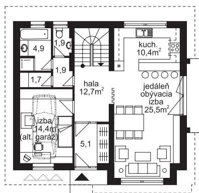
prízemie
