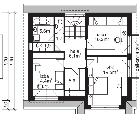
podkrovie
