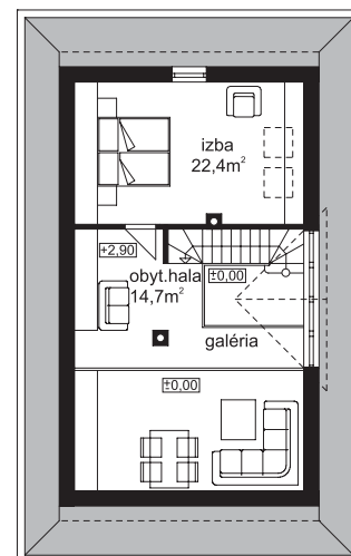
podkrovie
