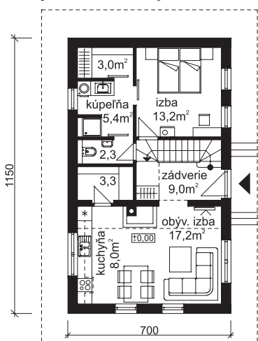
prízemie
