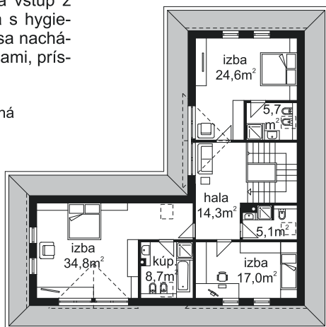
podkrovie
