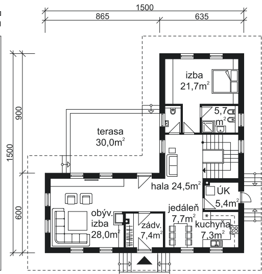
prízemie
