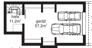
suterén
