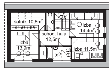
podkrovie
