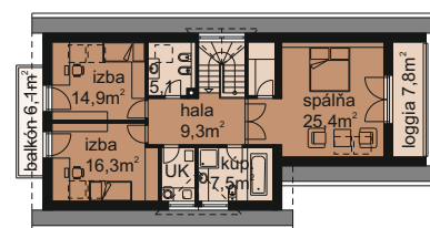
podkrovia
