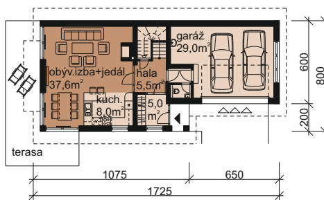
prízemie
