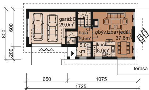
prízemie
