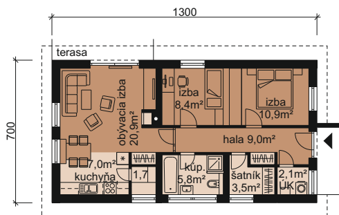
prízemie
