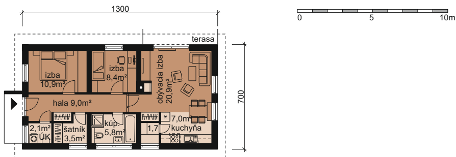
prízemie
